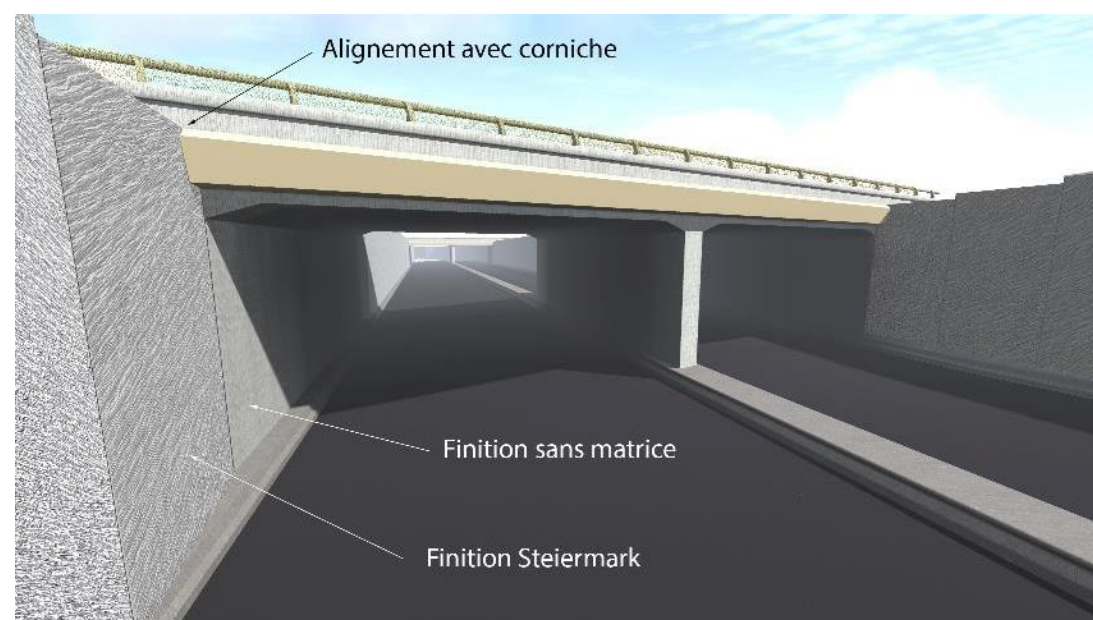
Figure 26 : trémie ouverte avec murs de soutènement
