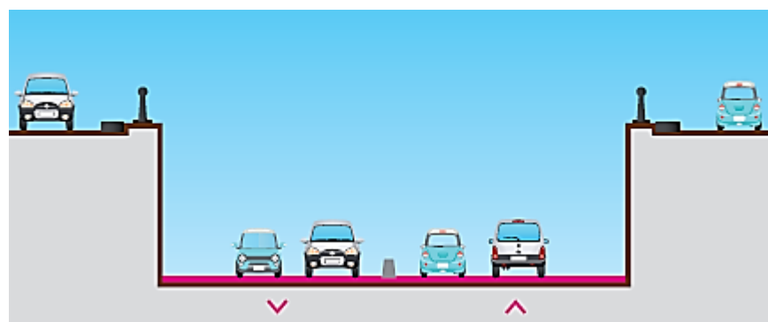
Figure 13 : Profil en travers type de la section sud de la partie centrale
